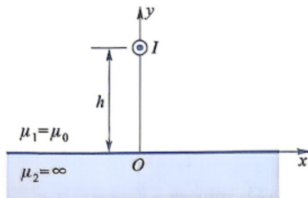
图 3.5.24 直线电流与 无限大铁板平面
