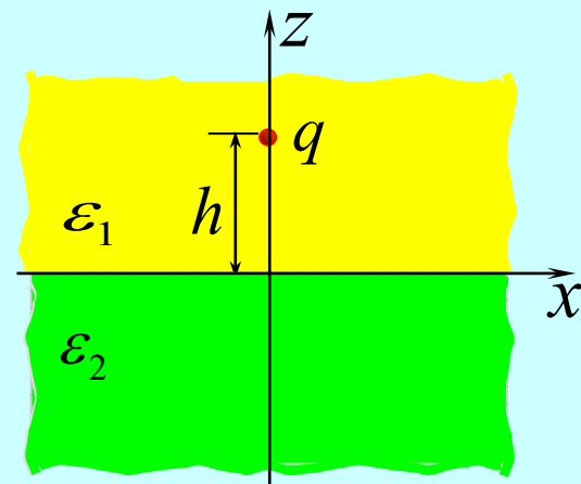
图1 点电荷与电介质分界面
