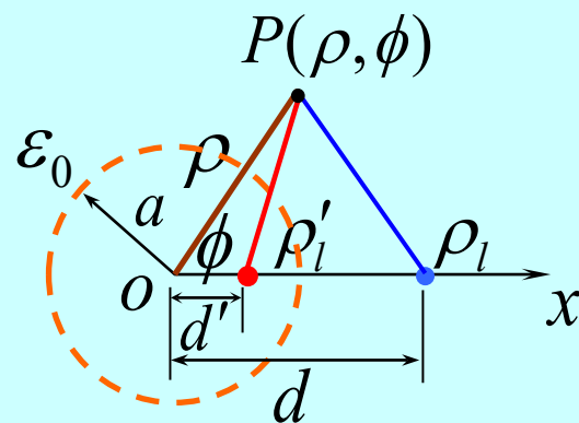
图2 线电荷与导体圆柱的镜像
