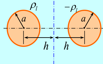
图1 两平行圆柱导体
