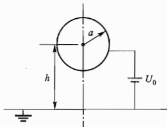
图 3.5.16 平行于地面的 圆柱导线
