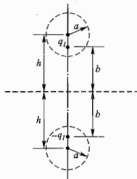
图 3.5.17 平行于地面的圆 柱导线的镜像
