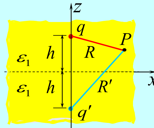
图2 介质1的镜像电荷
