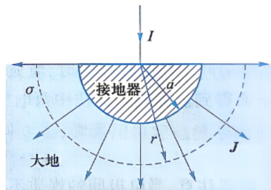
图 3.2.3 半球形接地器
